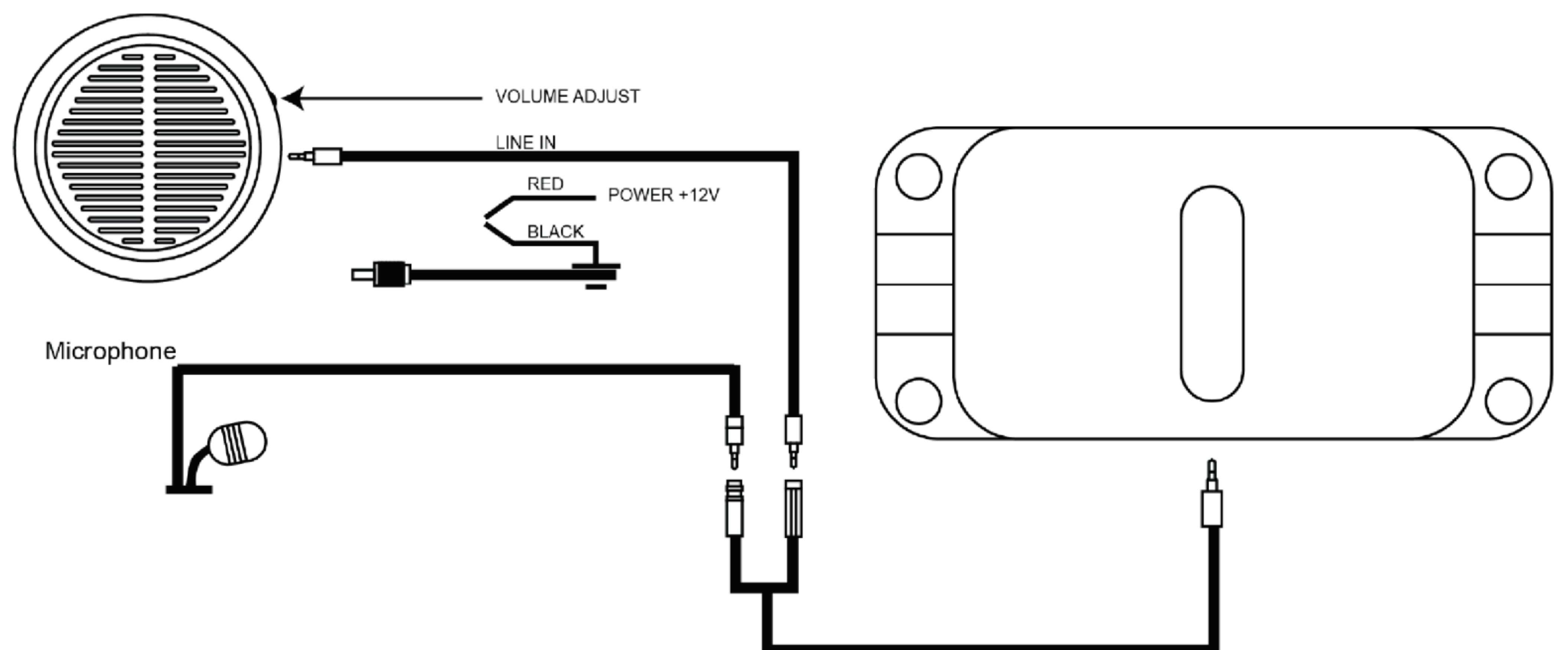
HFK Wiring Diagram
